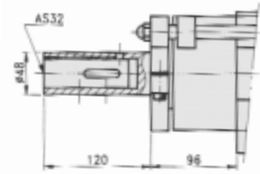
FD7-150-AS32
