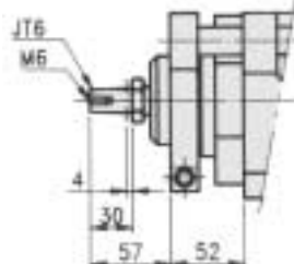
FD56-100-JT6
