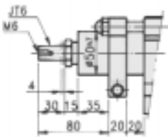
F6N-60-JT6
