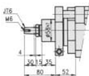
FD56-100-JT6 Multi
