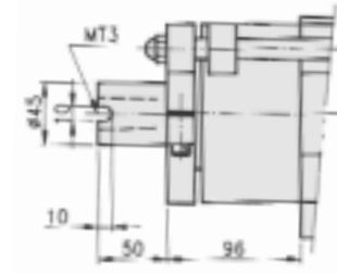
FD7-150-MT3B
