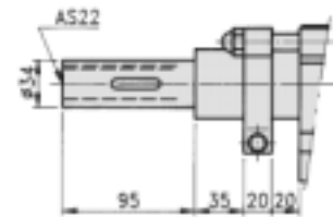
F6N-60-AS22
