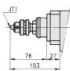
FD3-80-JT1
