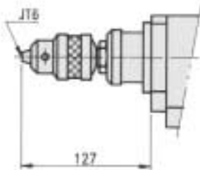
FD55-80-JT6
